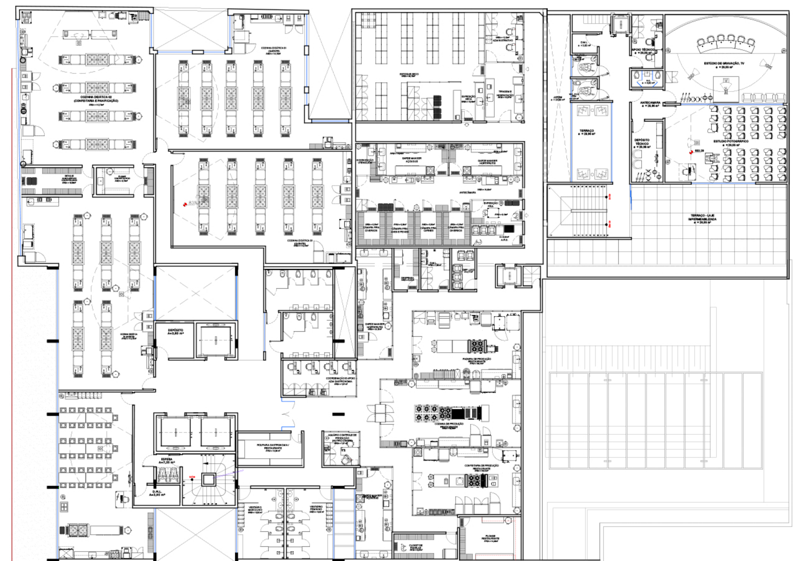
1º PAVIMENTO
