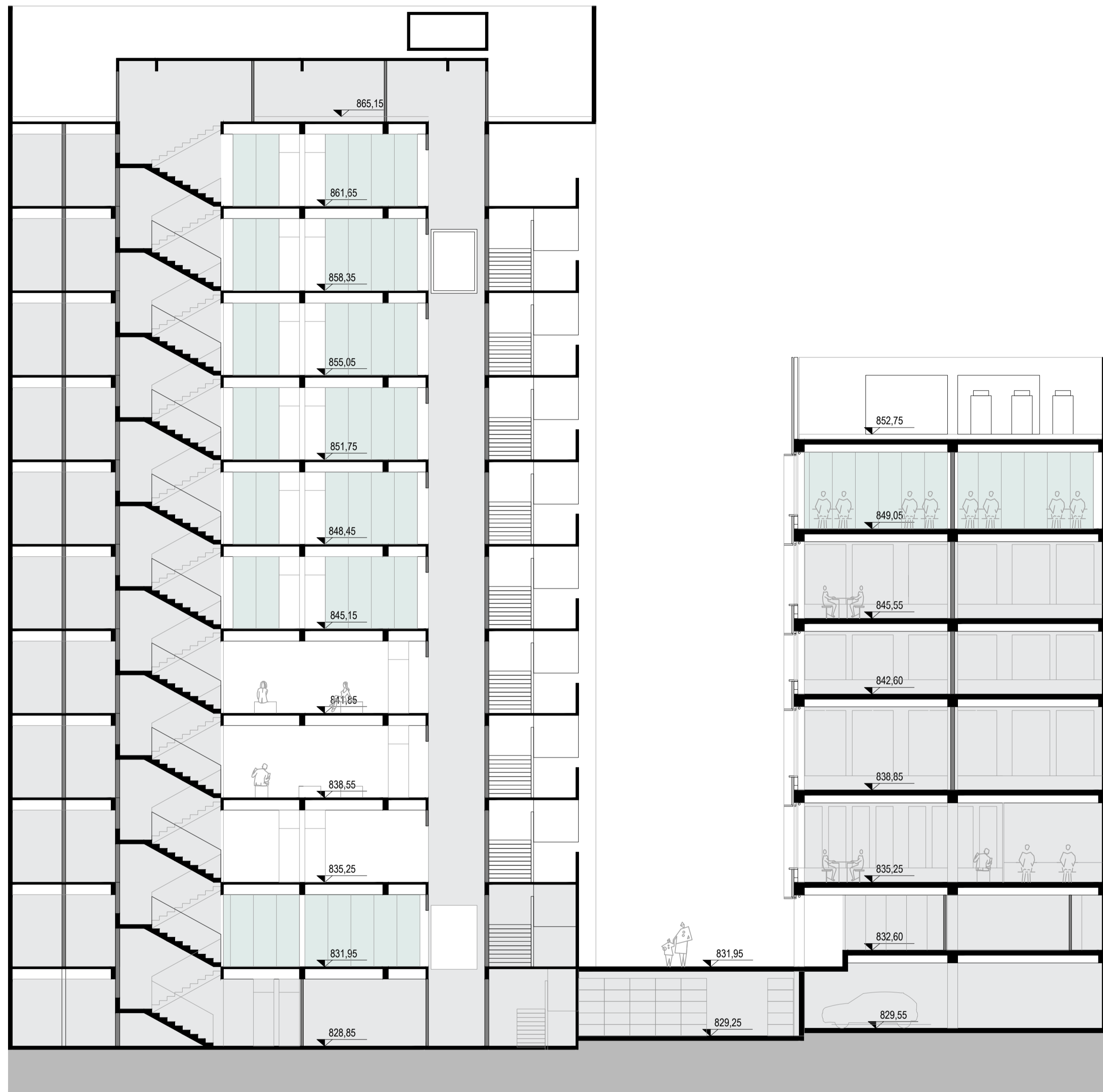
CORTE D esc 1:125
