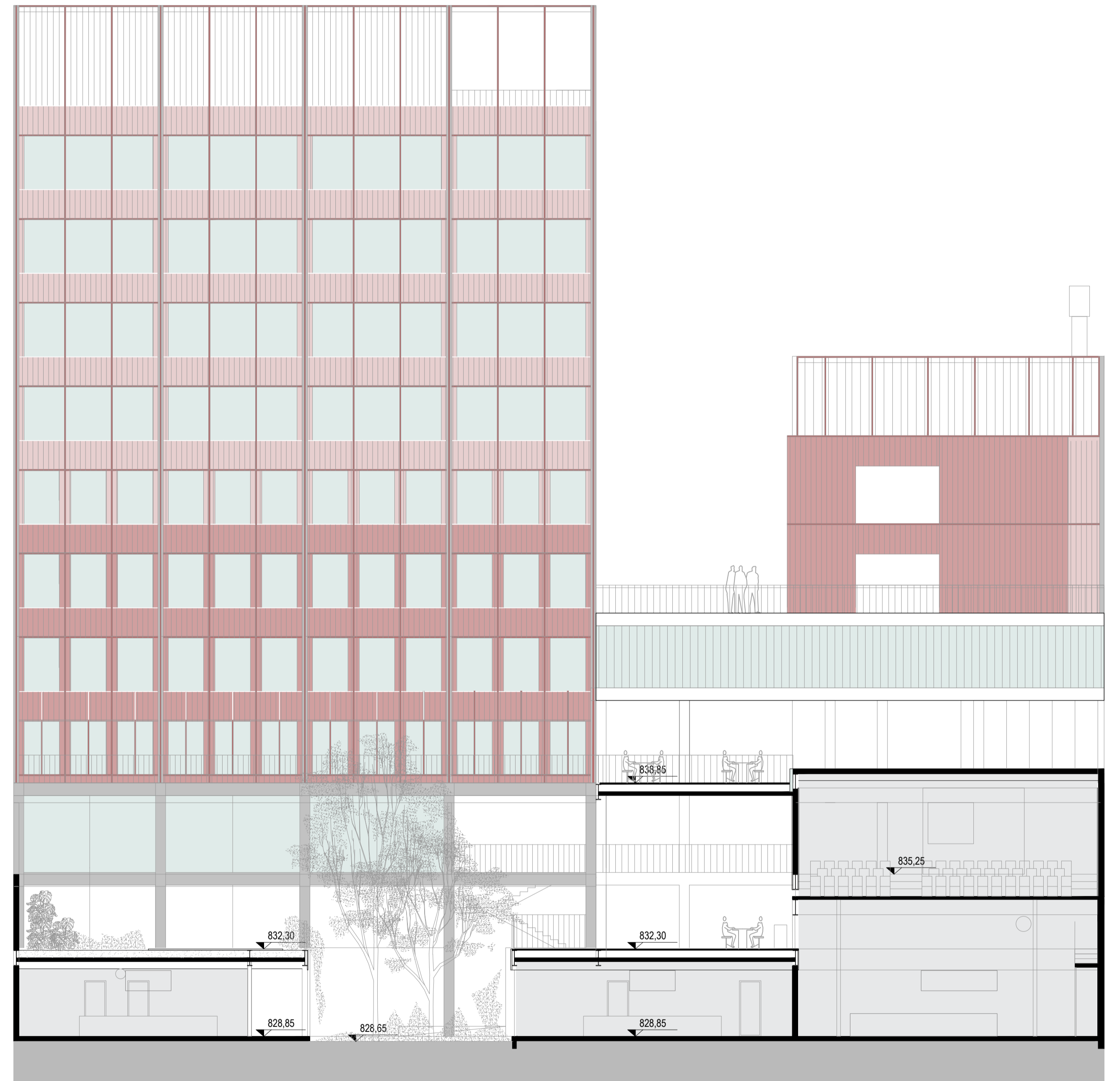
CORTE E esc 1:125
