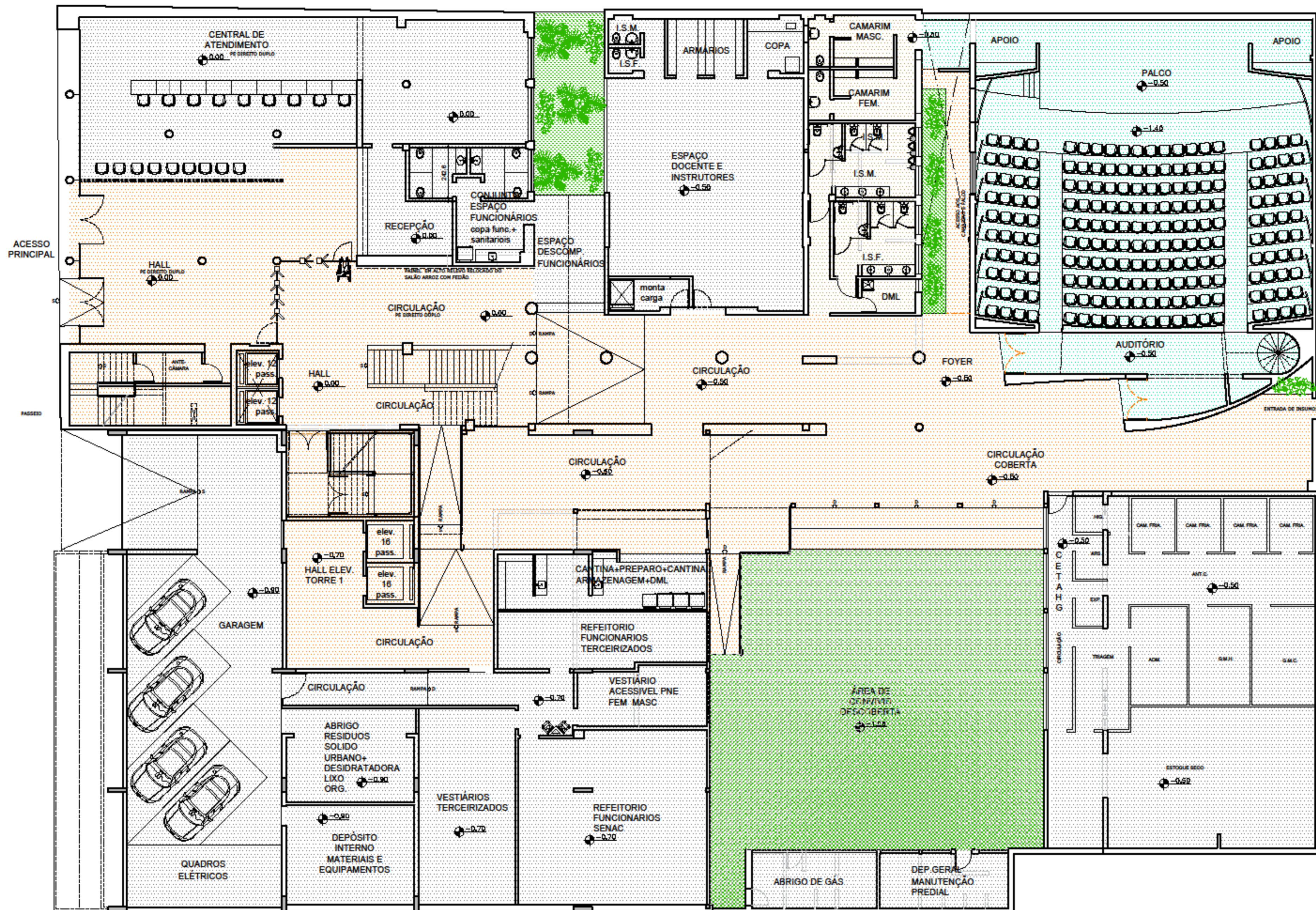
PLANTA - BLOCO 1_SUBSOLO - BLOCO 2_TÉRREO
