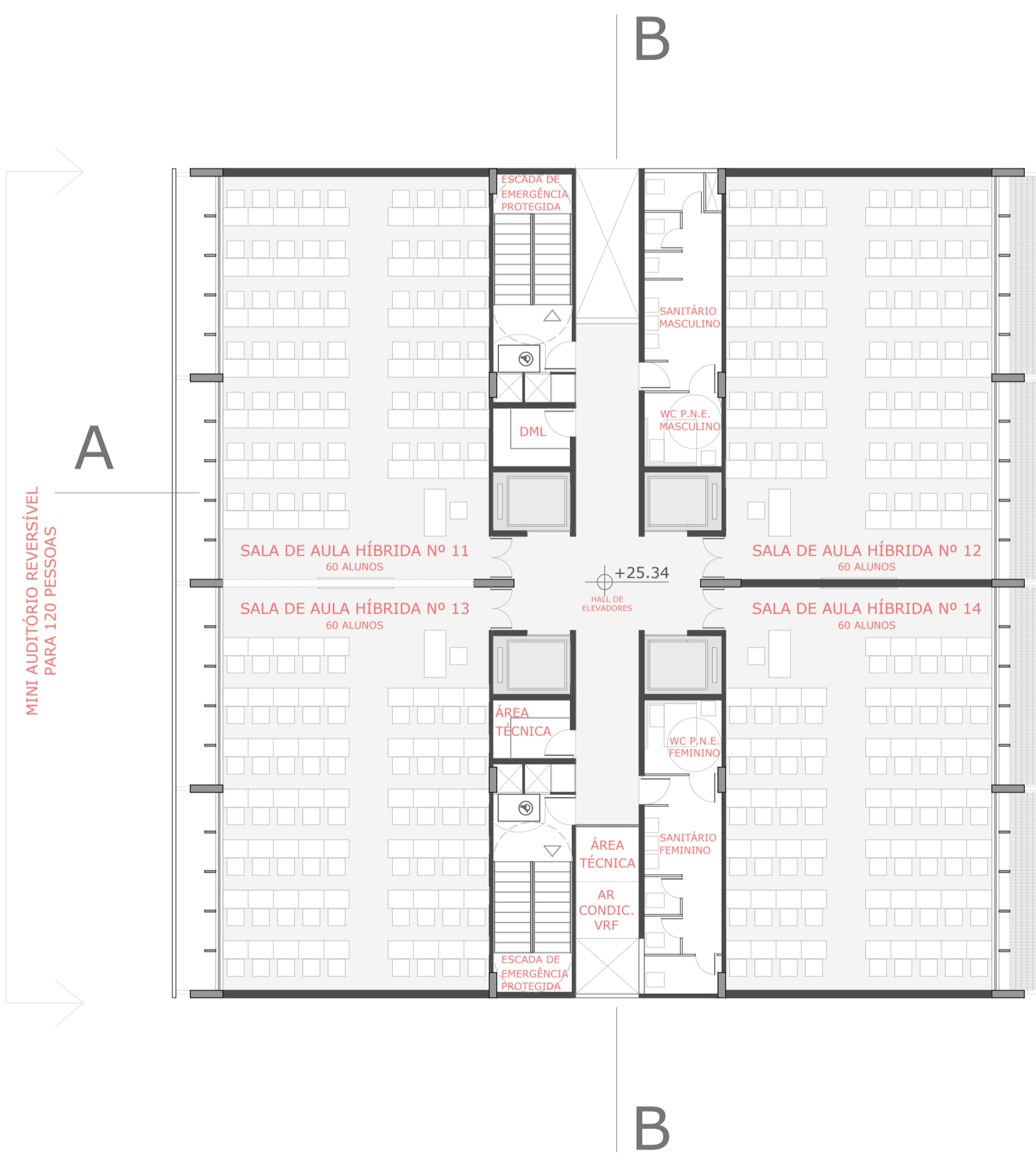
7º, 8º E 9º PAVIMENTO ESCALA 1:125
