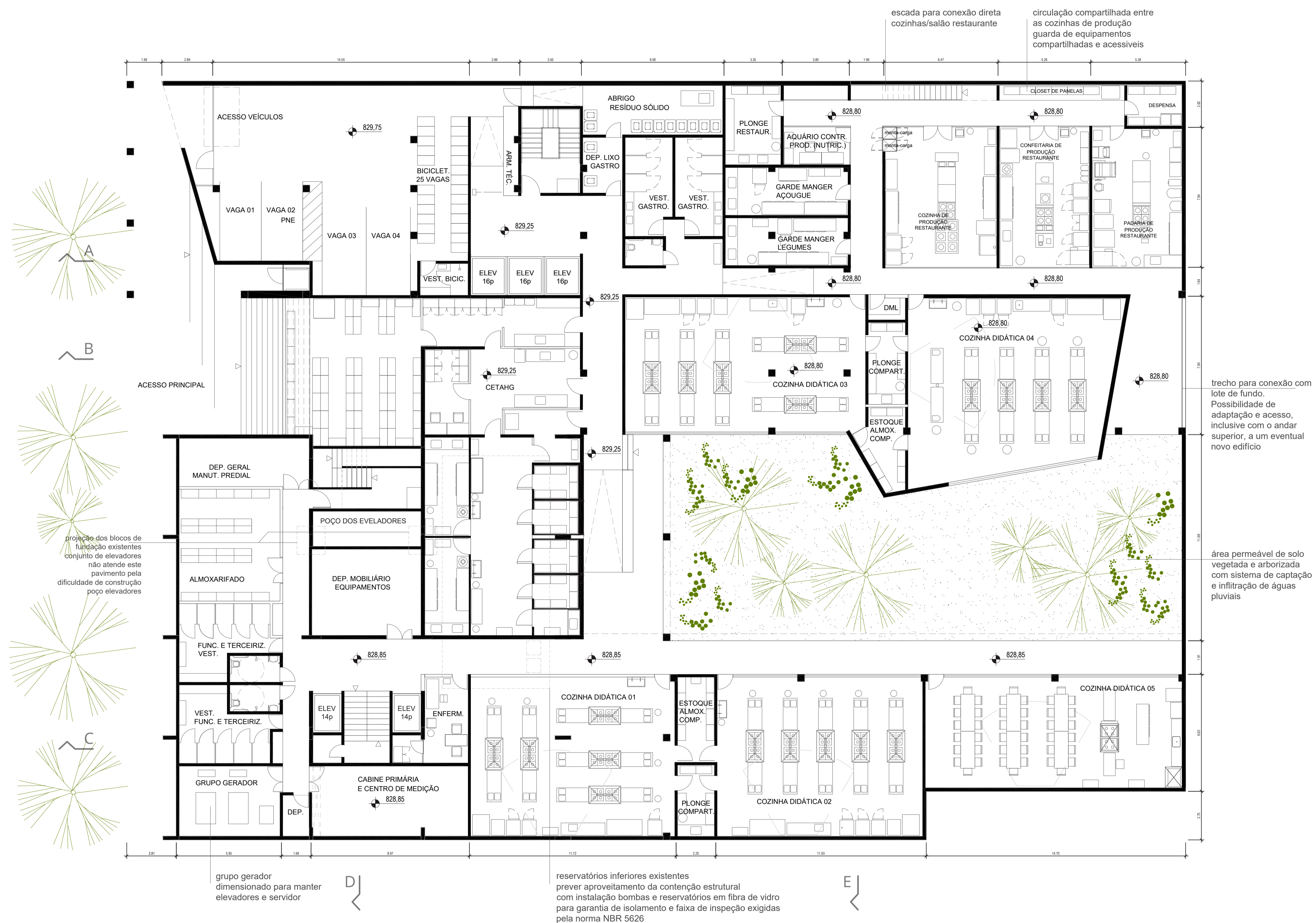
PLANTA SUBSOLO esc 1:125
