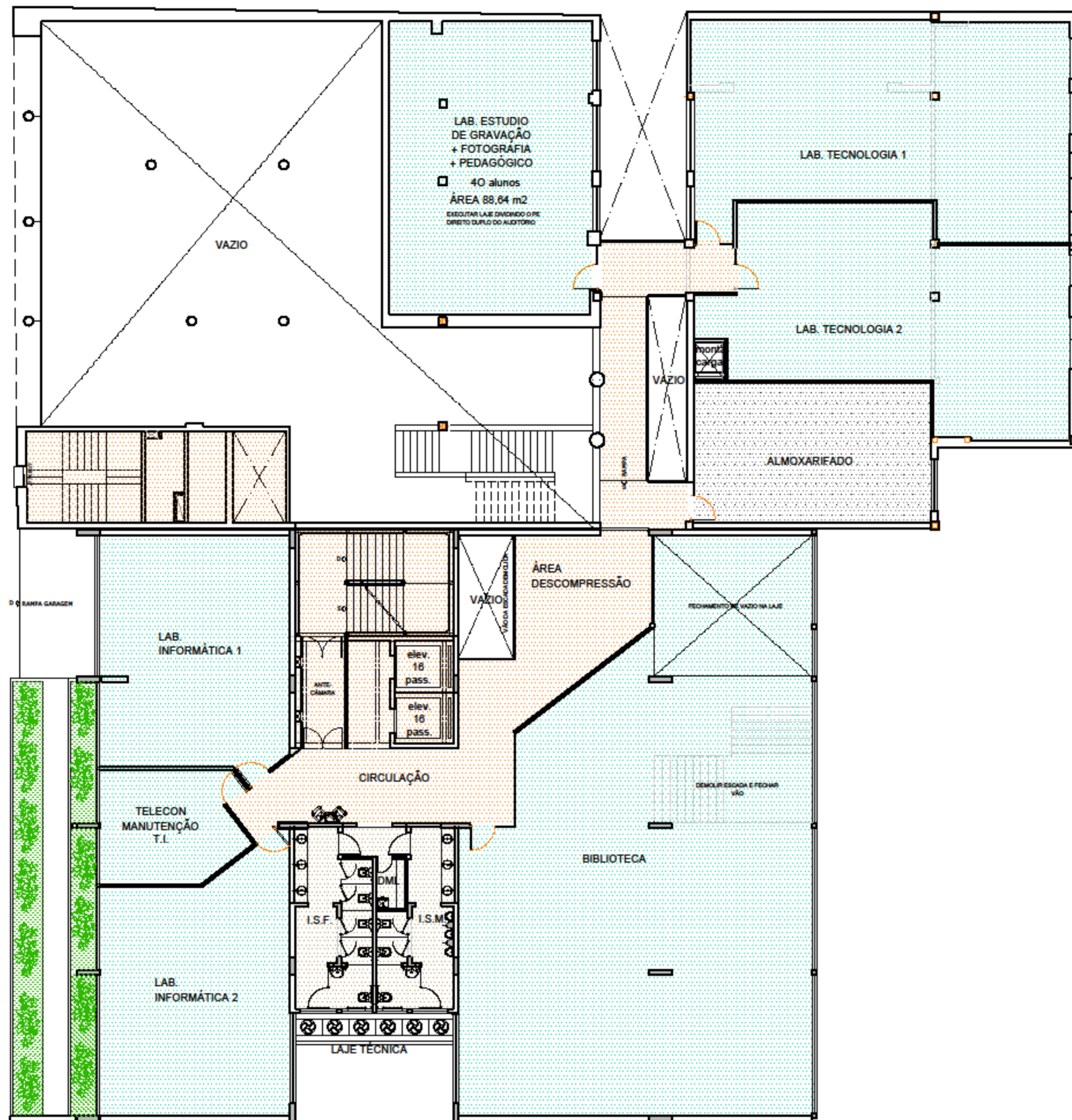
PLANTA - BLOCO 1_TÉRREO - BLOCO 2_SOBROLOJA escala 1/125 ÁREA CONSTRUÍDA: 1.085,00m²
