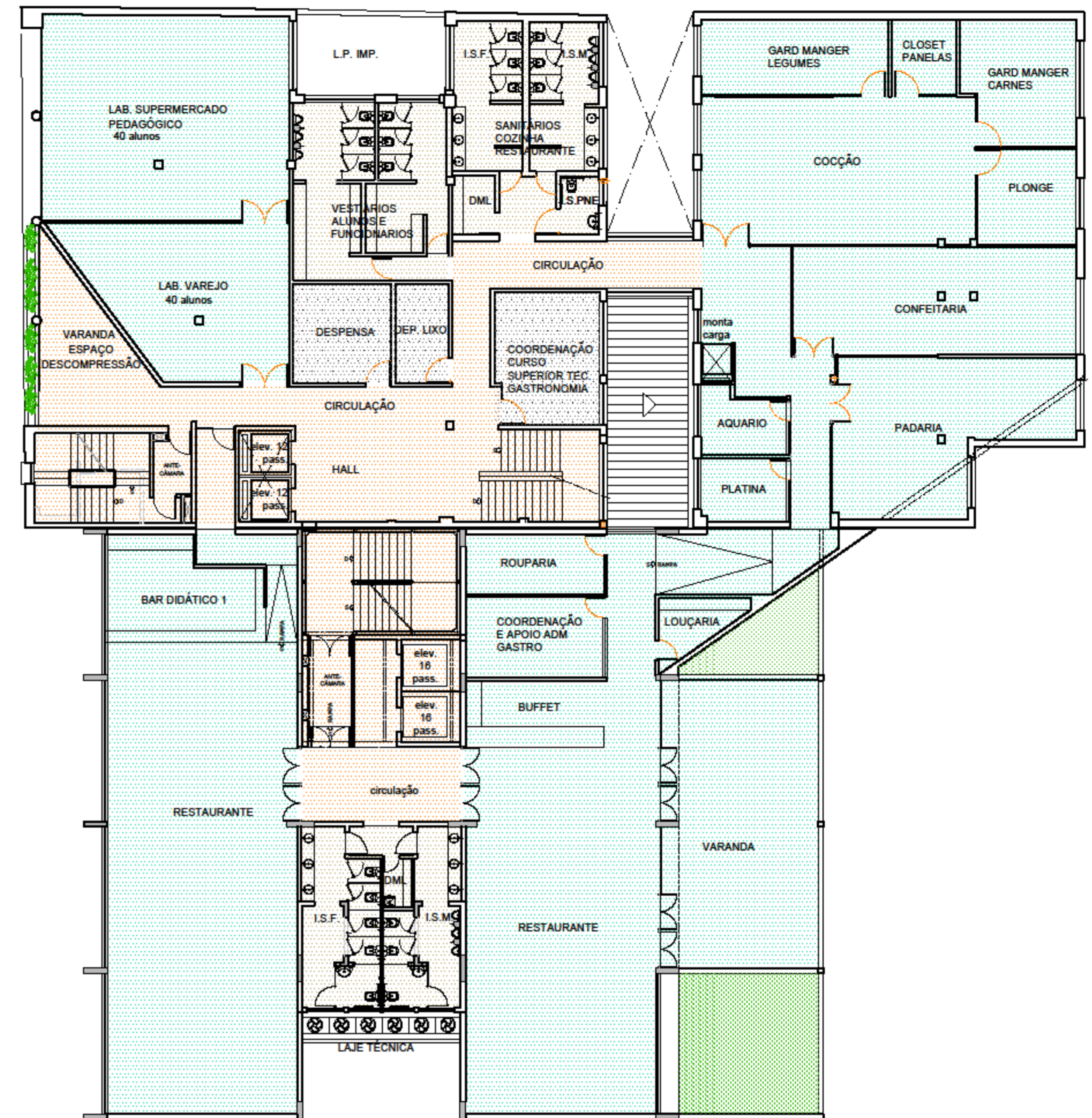
PLANTA - BLOCO 1 - BLOCO 2_1º PAVIMENTO escala 1/125 ÁREA CONSTRUÍDA: 1.225,00m²
