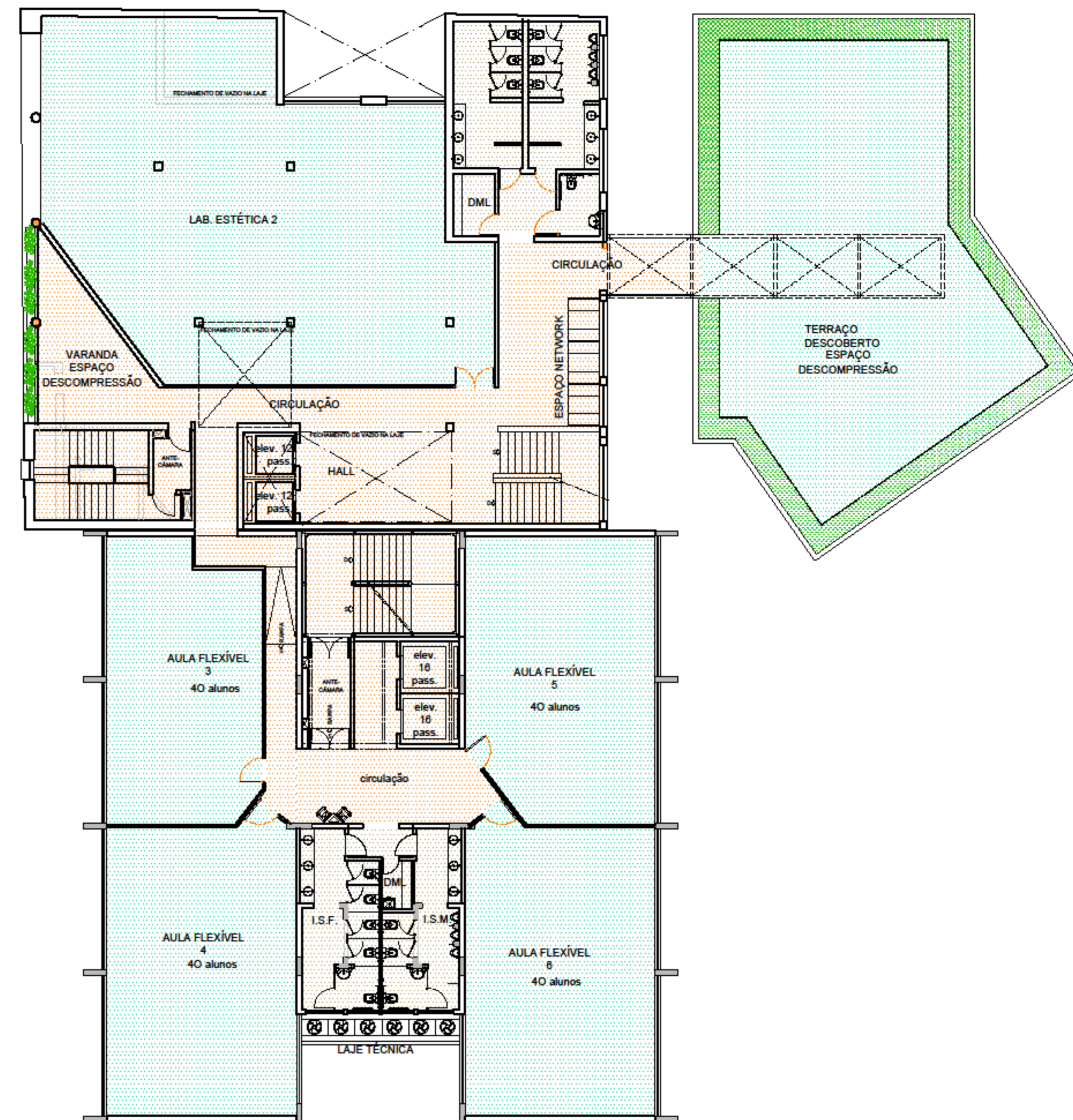
PLANTA - BLOCO 1 - BLOCO 2_5º PAVIMENTO escala 1/125 ÁREA CONSTRUÍDA: 905,00m²
