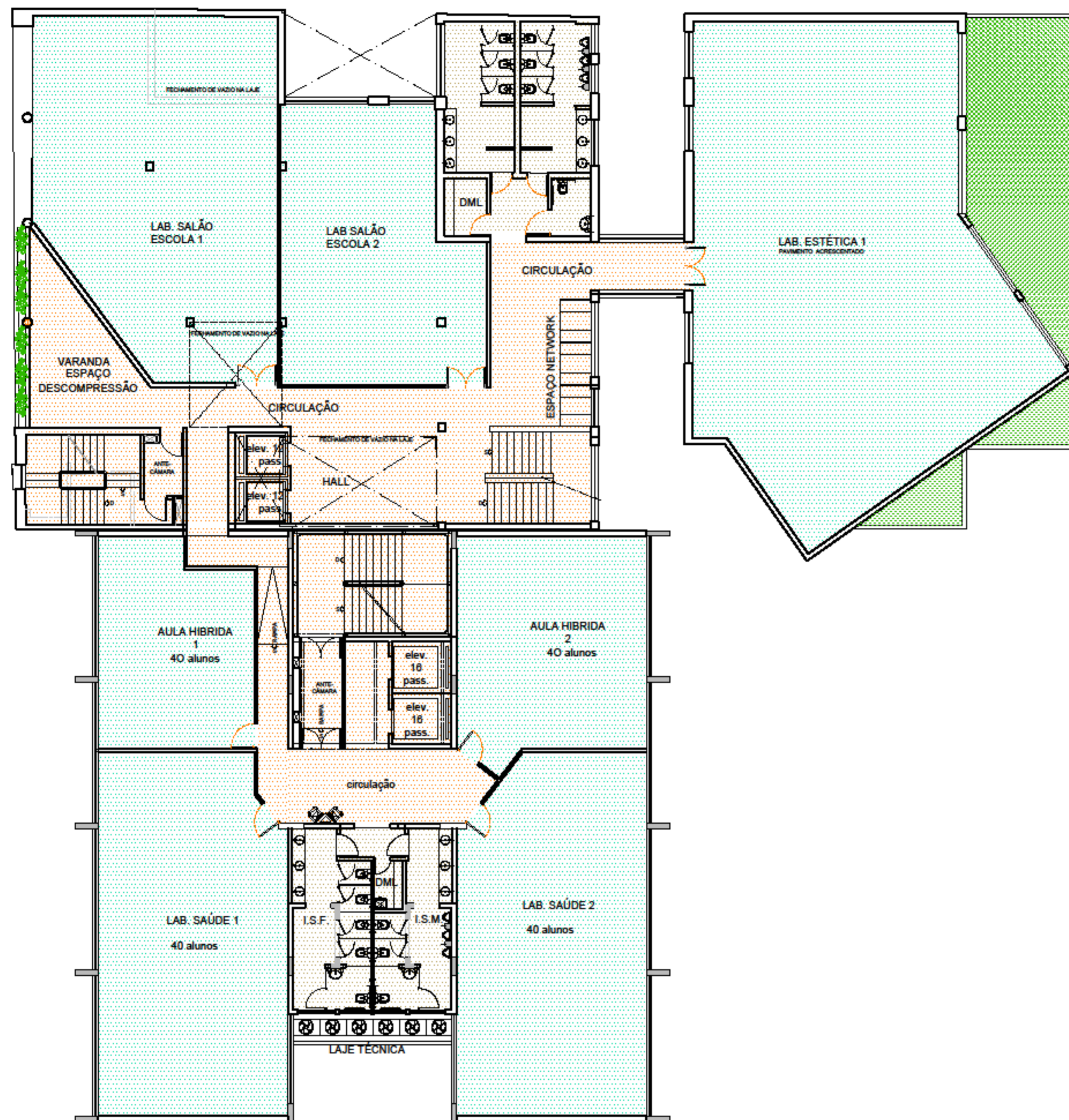
PLANTA - BLOCO 1 - BLOCO 2_4º PAVIMENTO escala 1/125 ÁREA CONSTRUÍDA: 1.135,00m²
